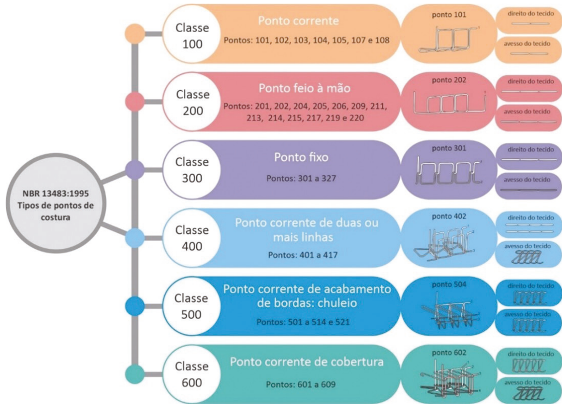
Figura VI 2: Classes e tipos de pontos de costura.
